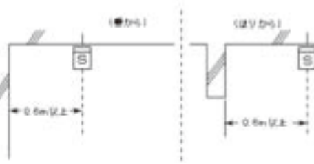
壁に設置する場合 ※天井から0.15m以上0.5m以内の位置にある壁
