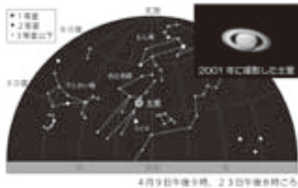
土星が見える星空と2001年に撮影した土星の写真。
