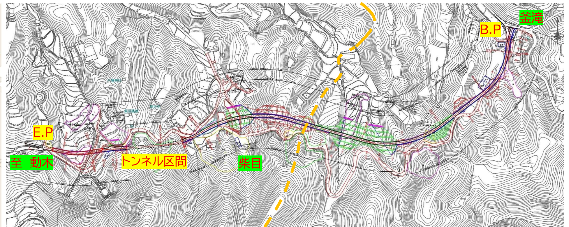
平面図
